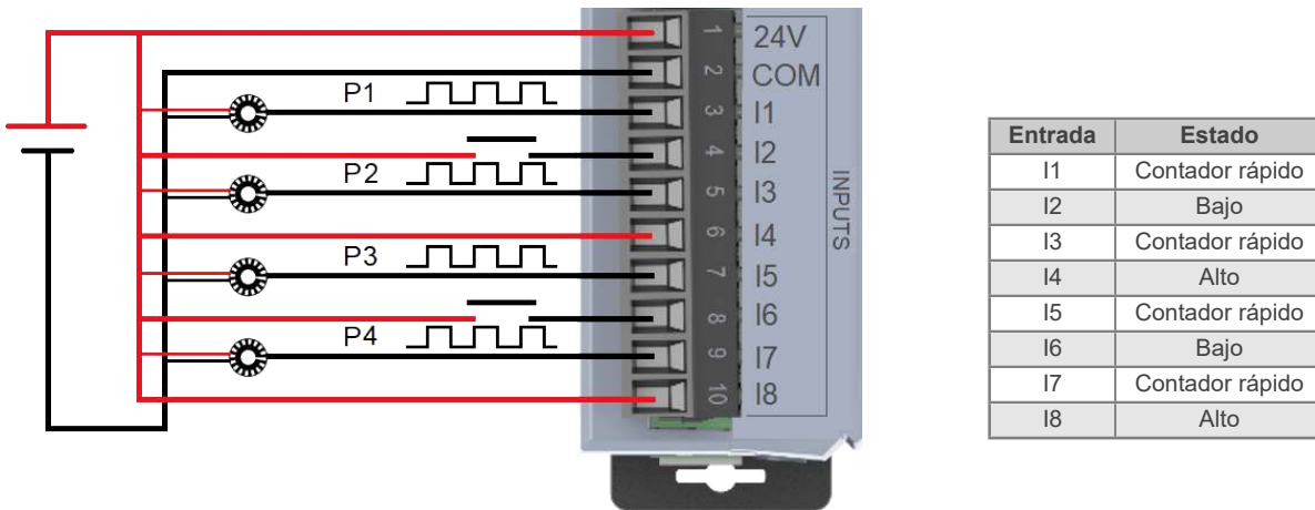
Figura 11.4: Función 4 - Configuración como contador rápido + entrada digital
